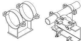
Rohr-Befestigungen, Rohr-Lager Rohr-Abhängungen (fest/gedämmt) Pipe fixings
