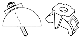
Schrägzug-Spannelemente/-Anker für Windverbände Kurvenstücke für Schrägzug bis 45° Angular tensile joints and anchors
